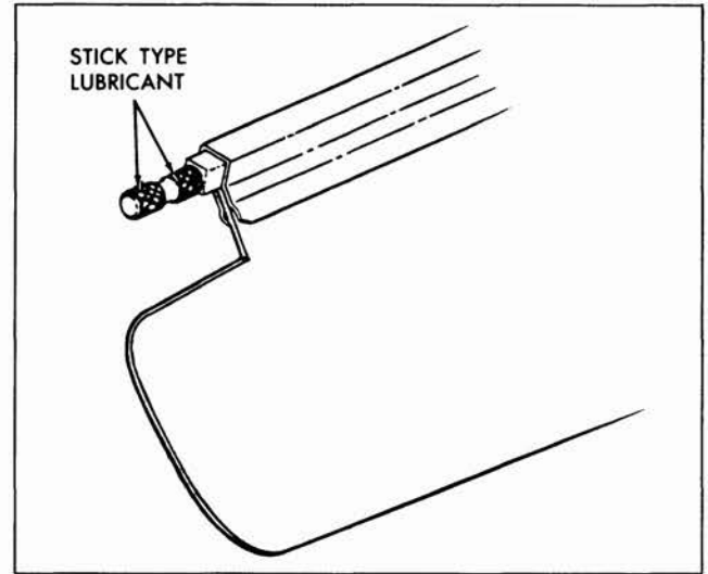
Fig. 10-7 Sunshade Rod
