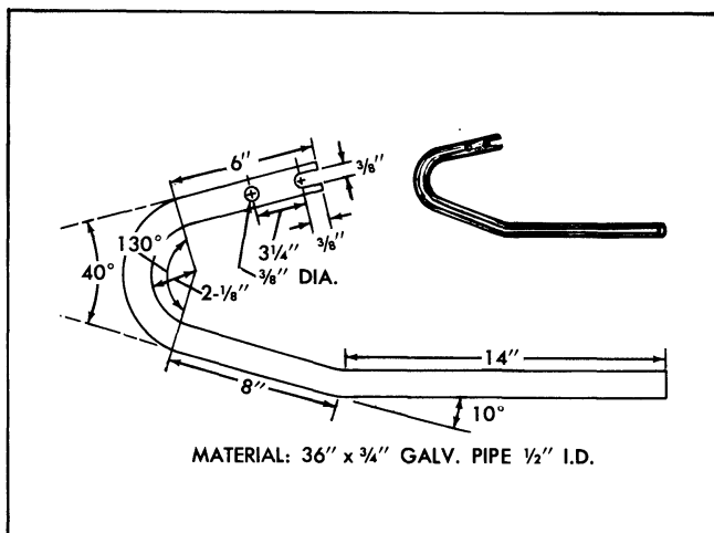
Fig. 15-7 Torque Rod Tool
