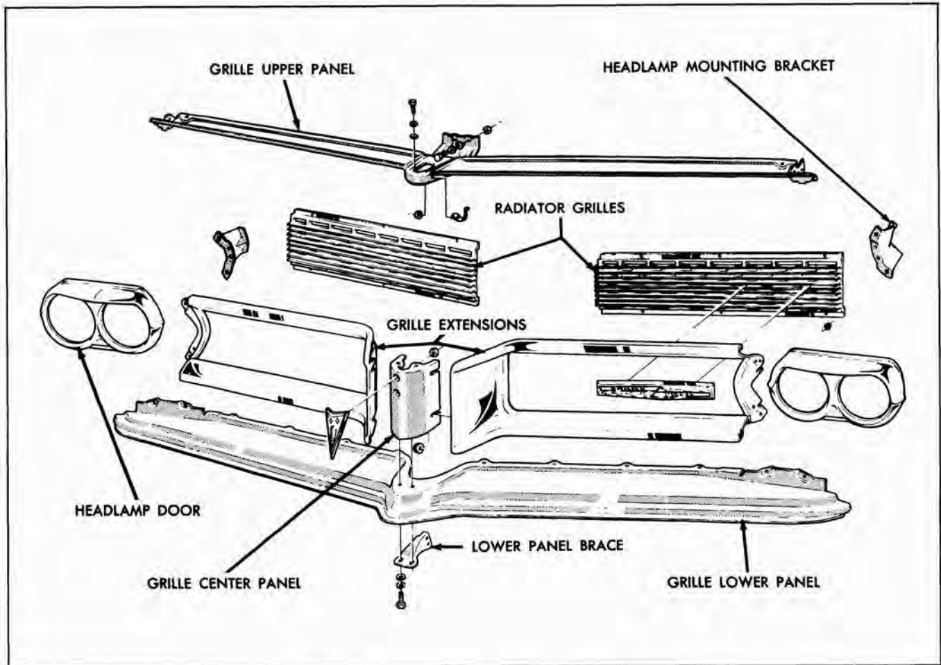
Fig. 1-13 Radiator Grille Assembly - Grand Prix
