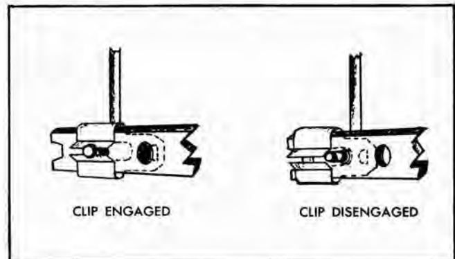
Fig. 13-11 Door Lock Spring Clip
