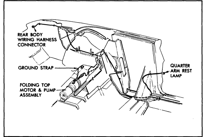
Fig. 19-5 Rear Body Wiring
