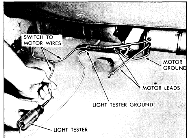
Fig. 22-66 Checking Motor Wiring
