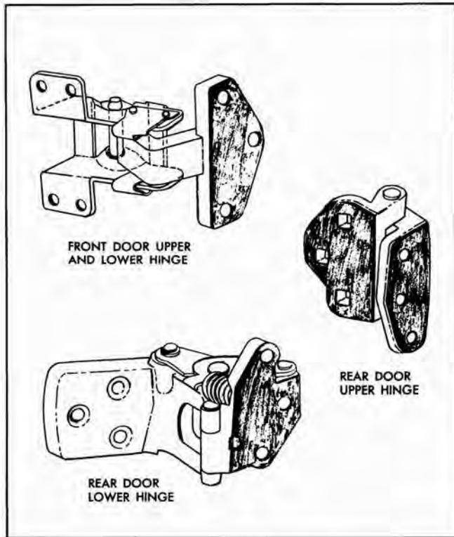
Fig. 13-14 Door Hinges
