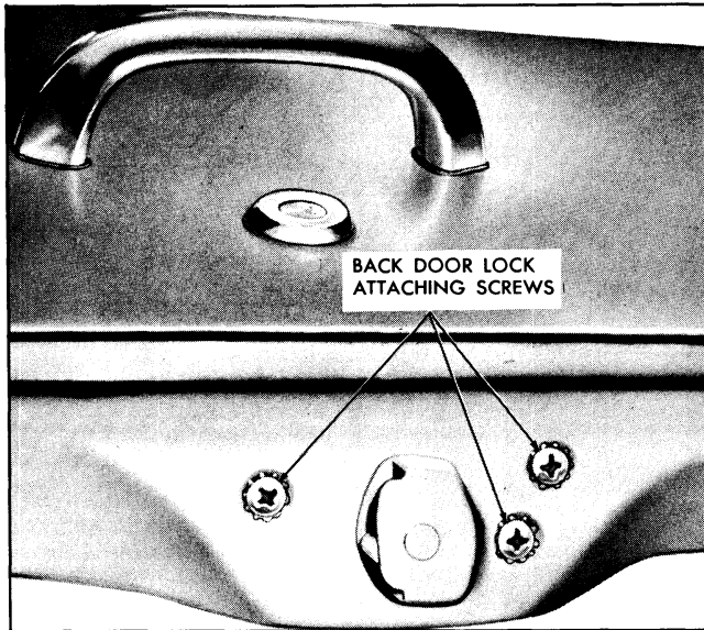
Fig. 15-15 Back Door Lock
