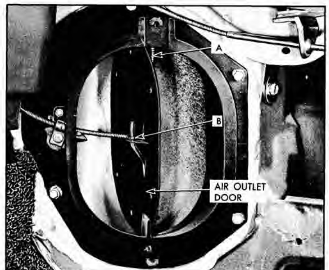
Fig. 2-13 Air Outlet Door
