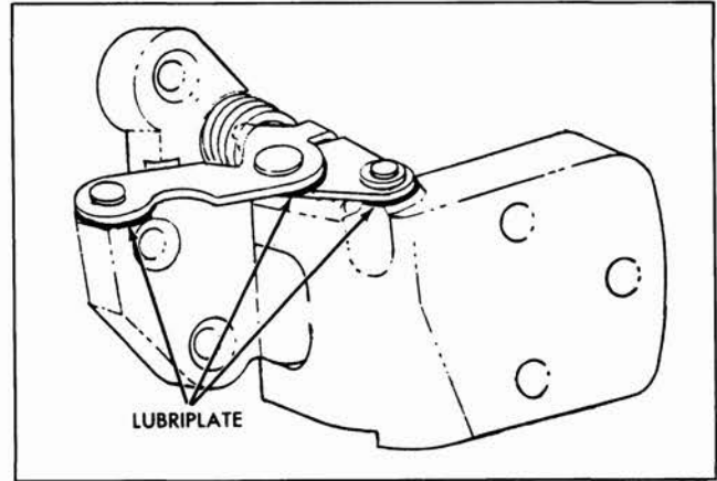
Fig. 10-4 Rear Door Hinge
