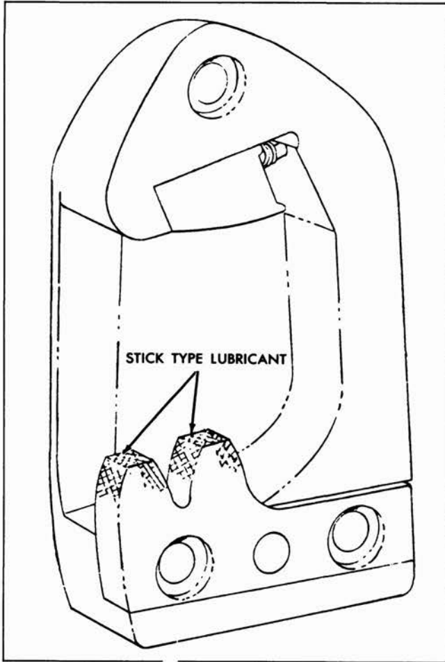
Fig. 10-2 Door Lock Striker
