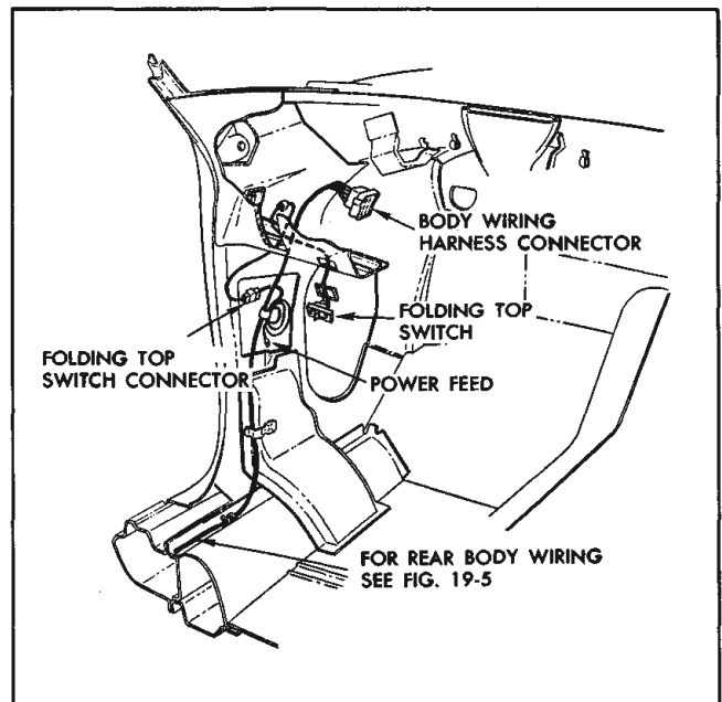
Fig. 19-4 Front End Wiring
