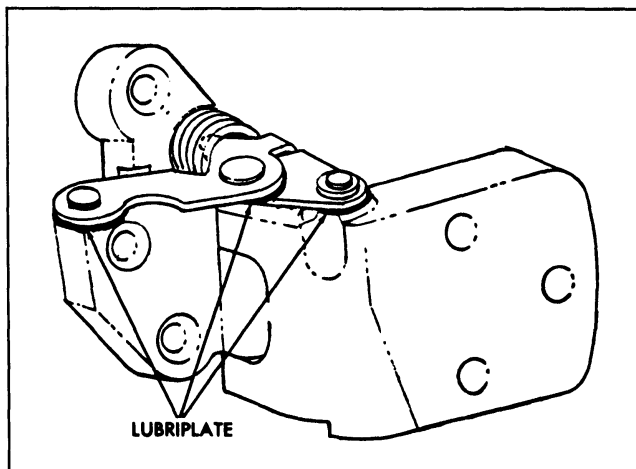
Fig. 20-4 Rear Door Hinge
