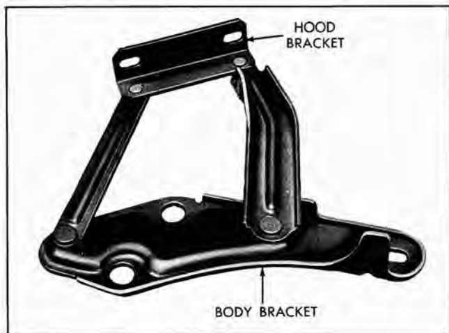
Fig. 11-3 Hood Hinge
