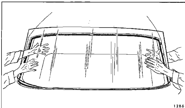
Fig. 4-7—Glass Installation
