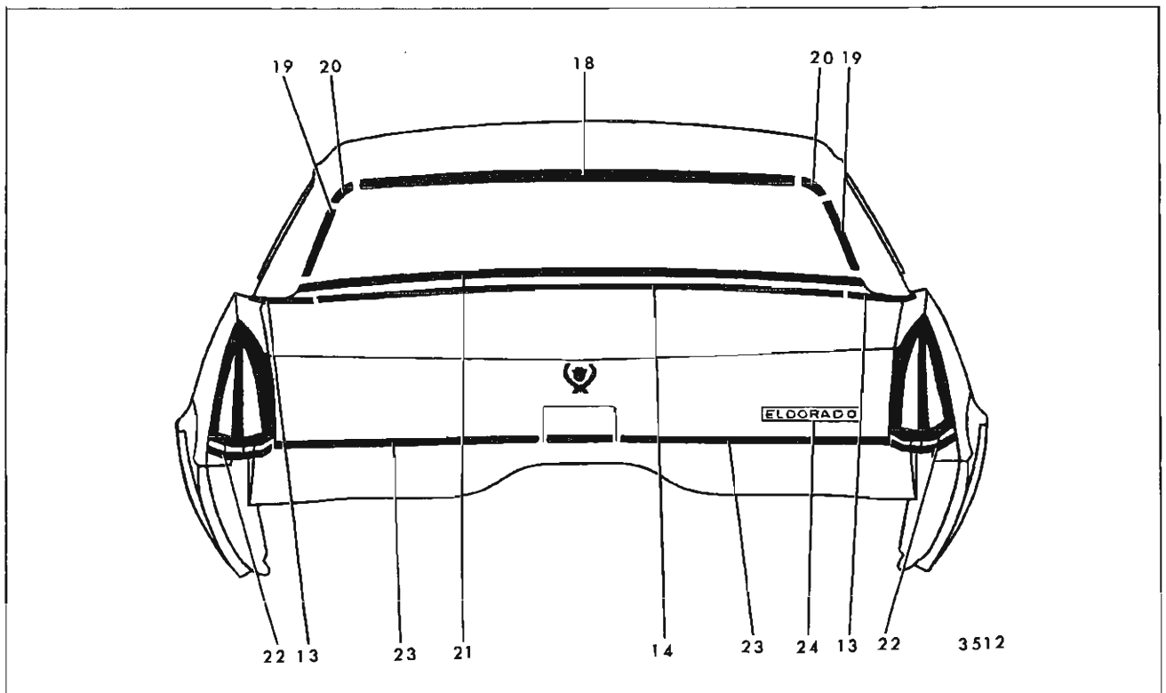
Fig. 17-100—Cadillac 69347 Styles
