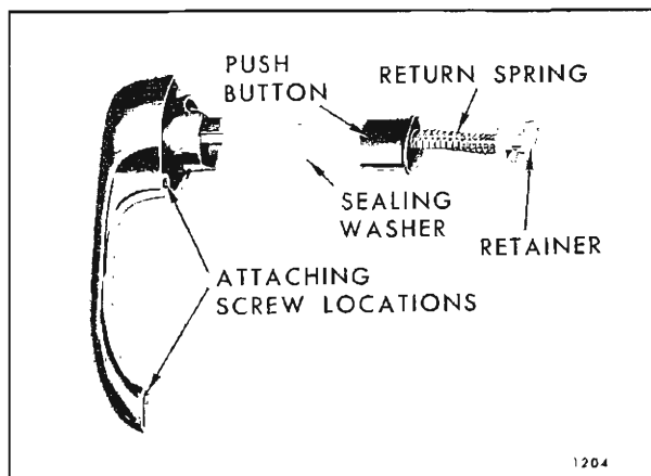
Fig. 6-23—Rear Door Outside Handle - All Styles
