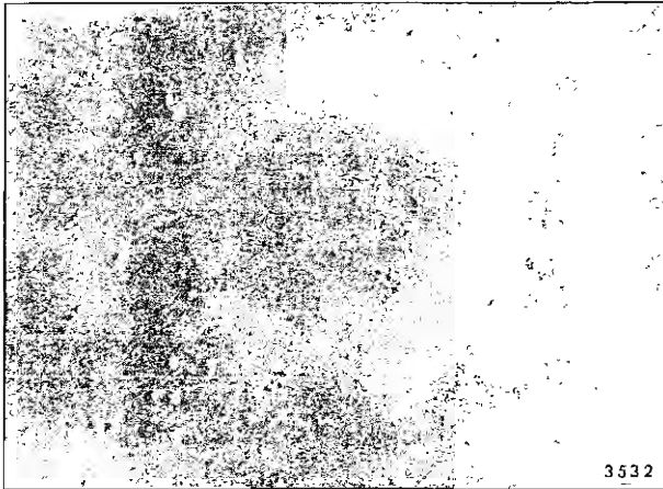
Fig. 1-20—Pinholing
