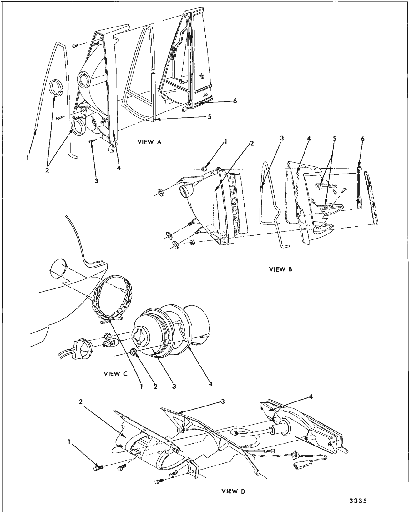
Fig. 16-45—Tail Lamp - Cadillac Styles
