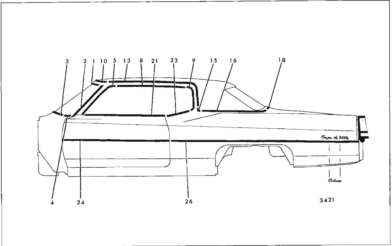
Fig. 17-92—Cadillac 68247-68347 Styles
