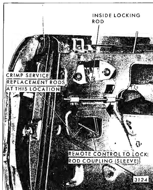
Fig. 6-65—Front Door Inside Locking Rod - Coupe Styles
