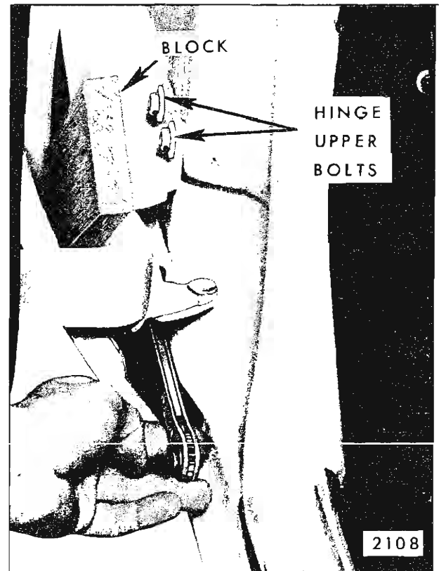
Fig. 6-63—Front Door Hinge Removal - "E" Styles
