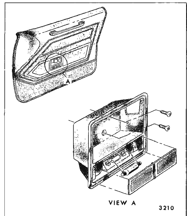
Fig. 14-4—Integral Door Arm Rest - Pontiac & Cadillac Styles
