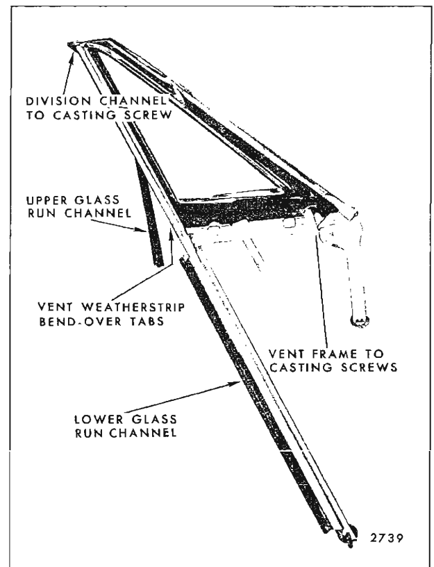
Fig. 6-73—Front Door Ventilator Assembly - "A-39" Styles
