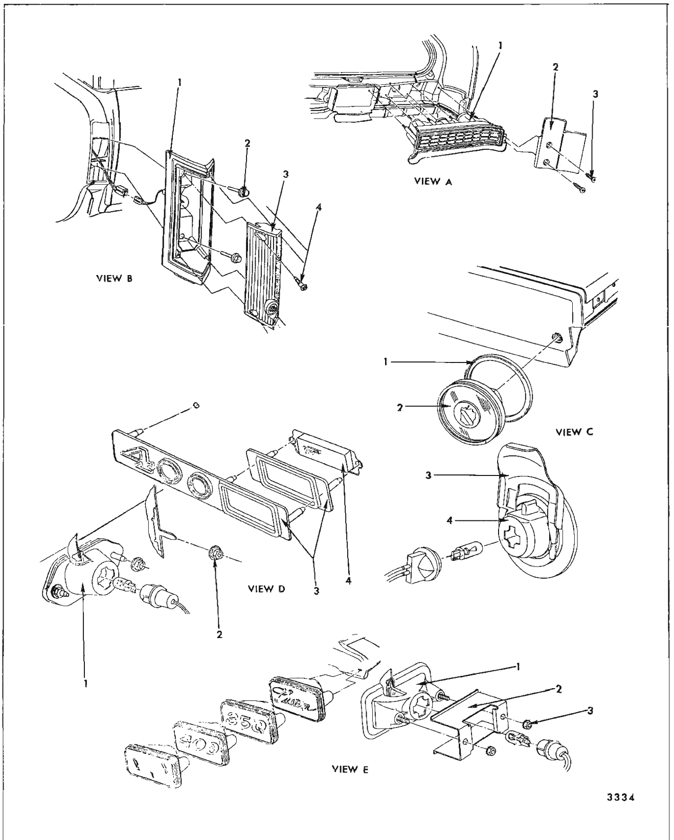
Fig. 16-44—Tail Lamp - Buick Styles
