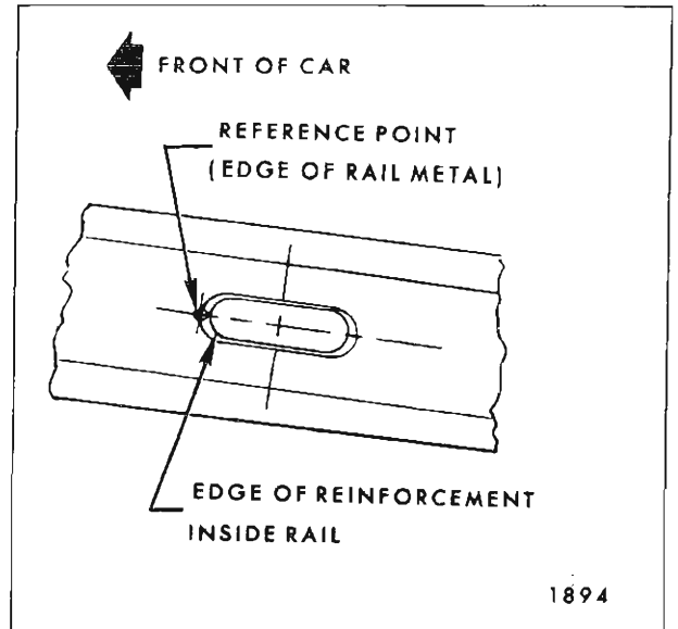
Fig. 3-3—Front Body Tie-Down Slot
