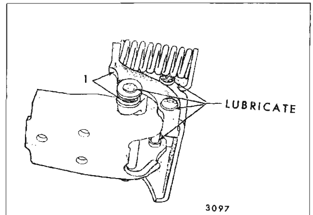
Fig. 2-3—"A-B & C" Styles Front Door Hinge Lubrication
