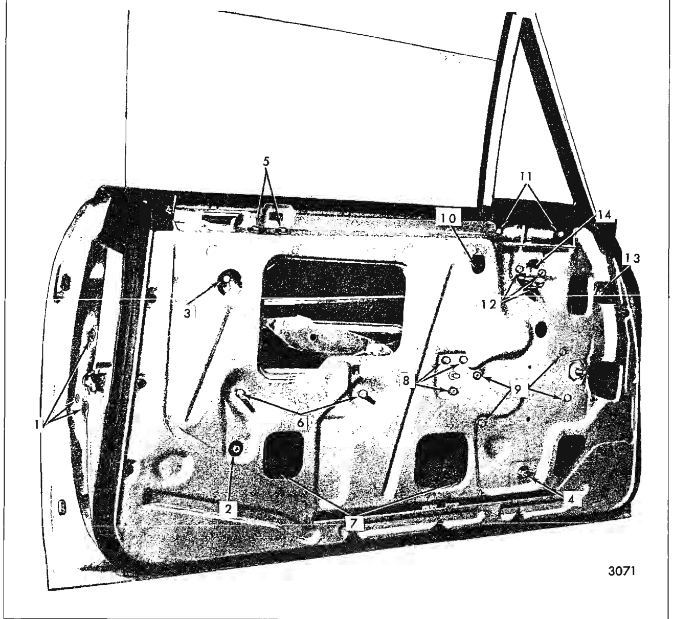
Fig. 6-40—Front Door Hardware - "A-39"
