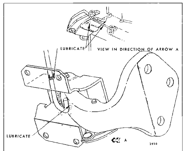
Fig. 2-4—"E" Body Front Door Hinge Lubrication
