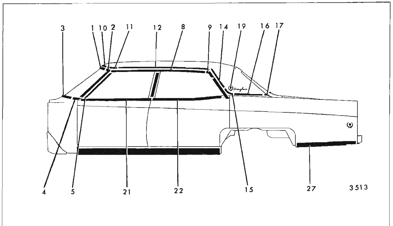
Fig. 17-95—Cadillac 68069-68169 Styles
