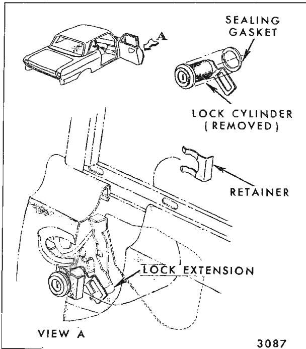
Fig. 6-68—Front Door Lock Cylinder Removal - All Styles
