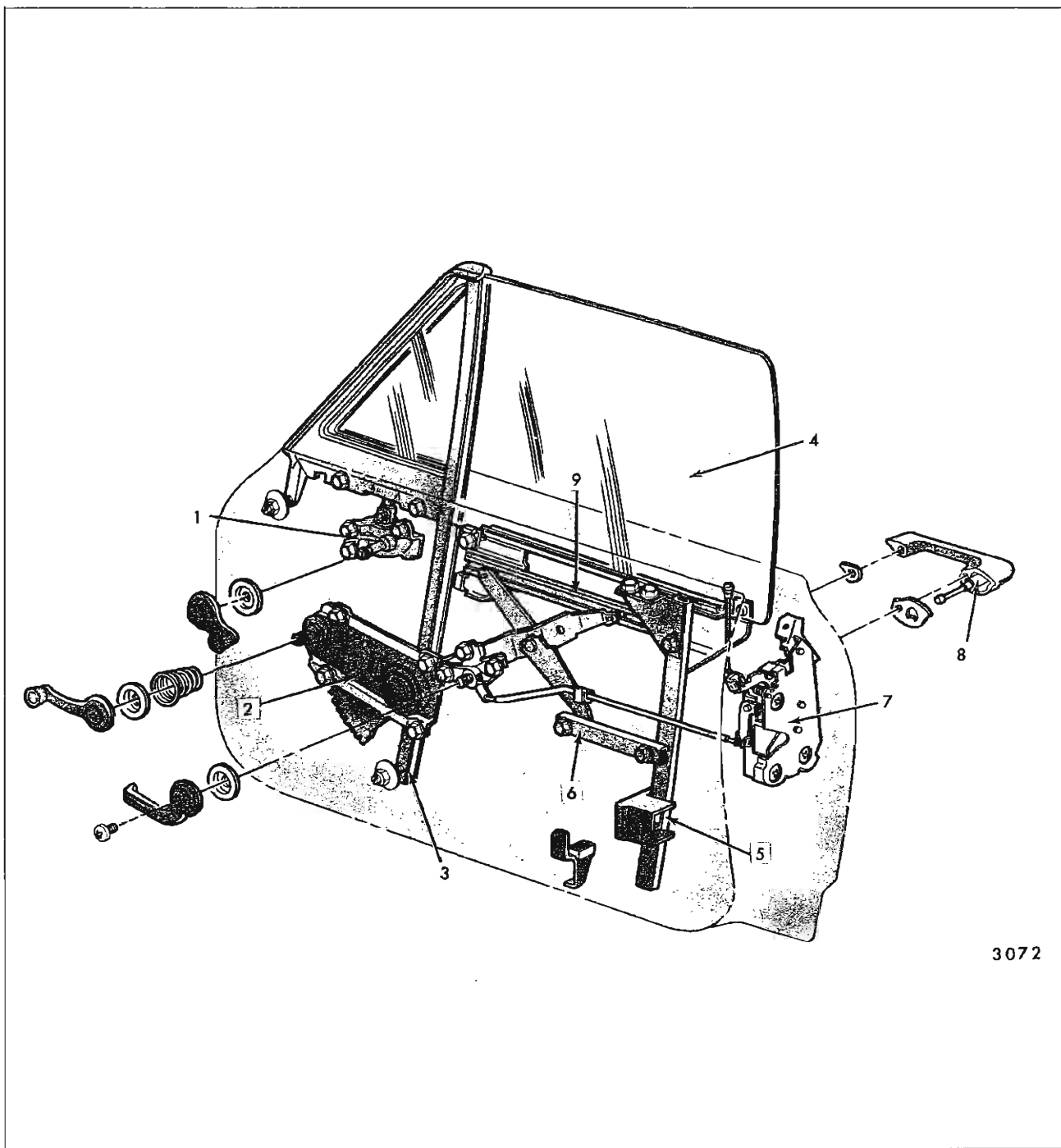
Fig. 6-39—Front Door Hardware - "A-39" Styles
