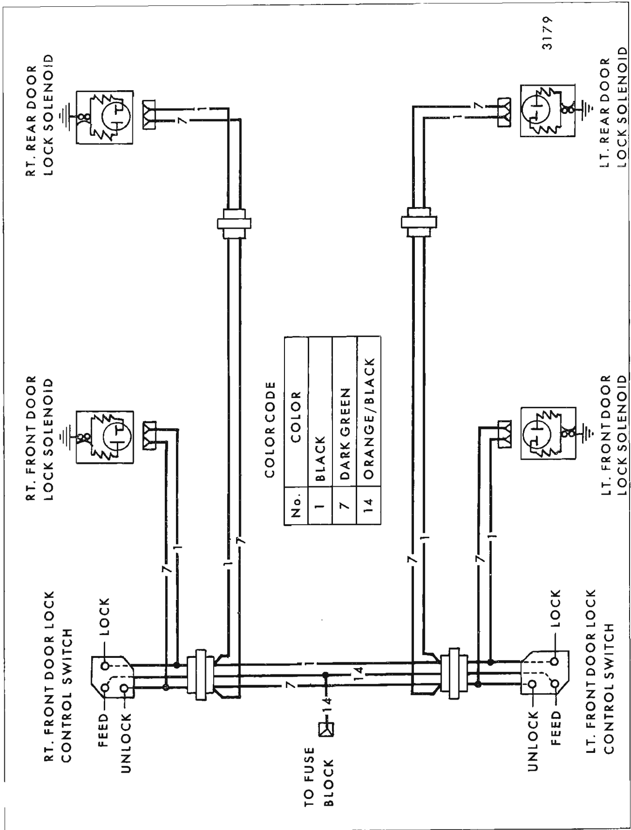
Fig. 16-49—Electric Door Lock Wiring Diagram
