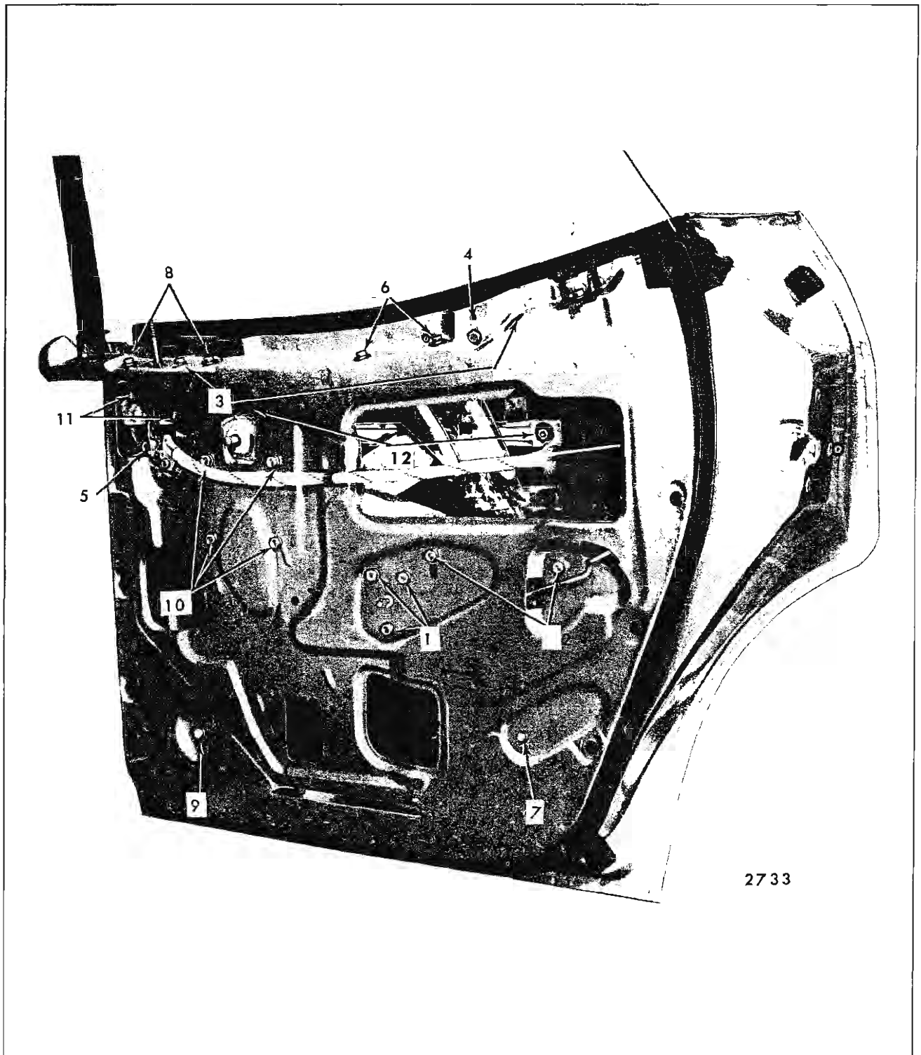
Fig. 6-108—Rear Door Hardware - "A-39" Styles
