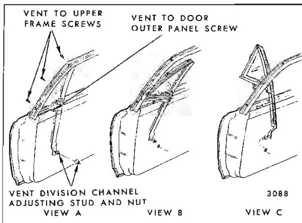
Fig. 6-74—Front Door Ventilator Removal
