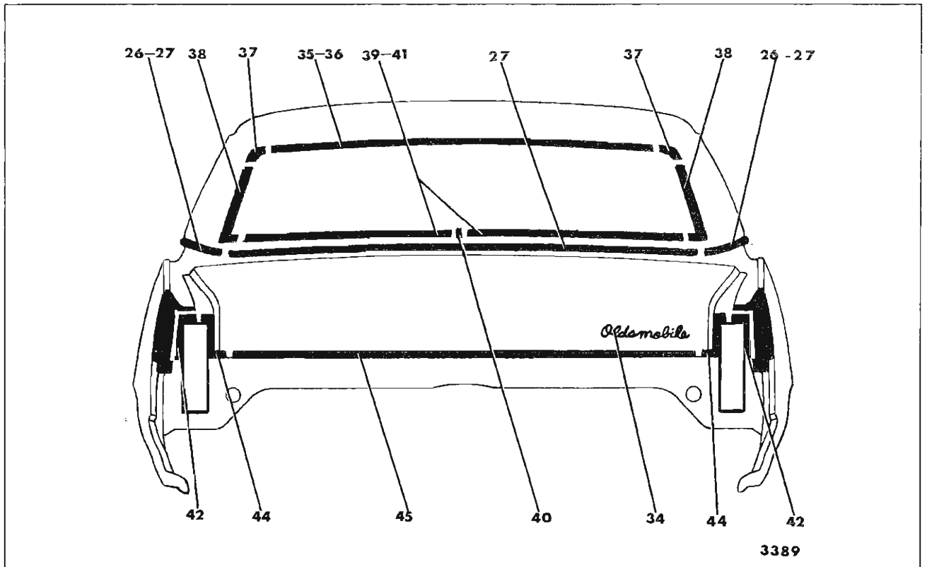
Fig. 17-71--Oldsmobile 38400-38600 Styles
